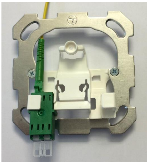
OptoUP Extensions inkl. 1x LC/APC Du-Adapter SM 1x Befestigungsplatte 1x1 (nicht im Set enthalten) 1x LC/APC Simplex Verbindungskabel (nicht im Set enthalten)
