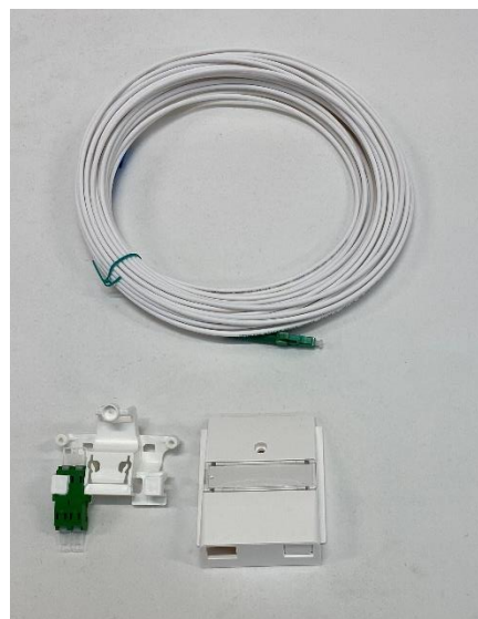
Extension pour OptoUP incl. 1 raccord Du LC/APC SM 1 câble de raccordement LC/APC Simplex de 15m
