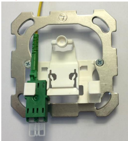
Extension OptoUP avec 1 raccord LC/APC Du SM 1 plaque de fixation 1x1 (non compris dans le set) 1 câble de raccordement LC/APC Simplex (non compris dans le set)
