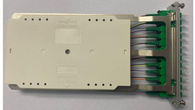
3HE/7TE Einschub mit 24x LC/APC spleissbereit eingelegt*
