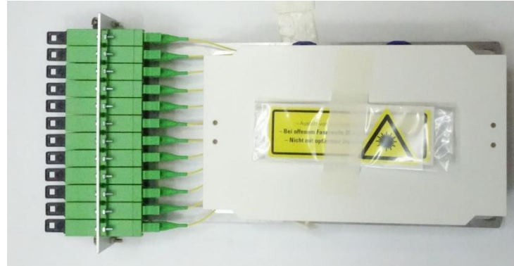
3HE/7TE Einschub mit 12x E-2000/APC spleissbereit eingelegt*
