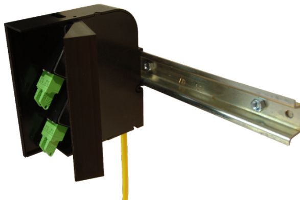
OptoC4 mit 4x E-2000/APC
